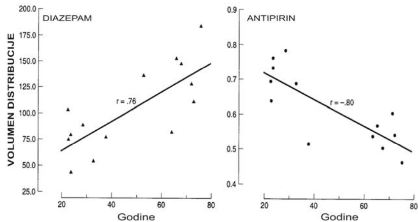
Slika 1. Promena u vrednosti volumena distribucije diazepam i antipirina sa godinama
