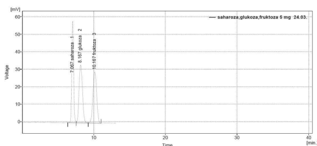
Slika 1. Hromatogram smeše standarda šećera
